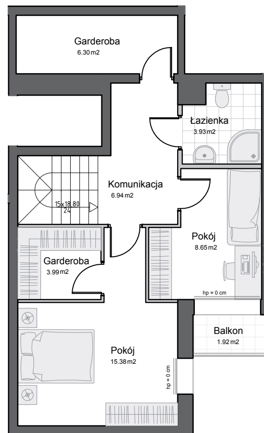
POZIOM 2
